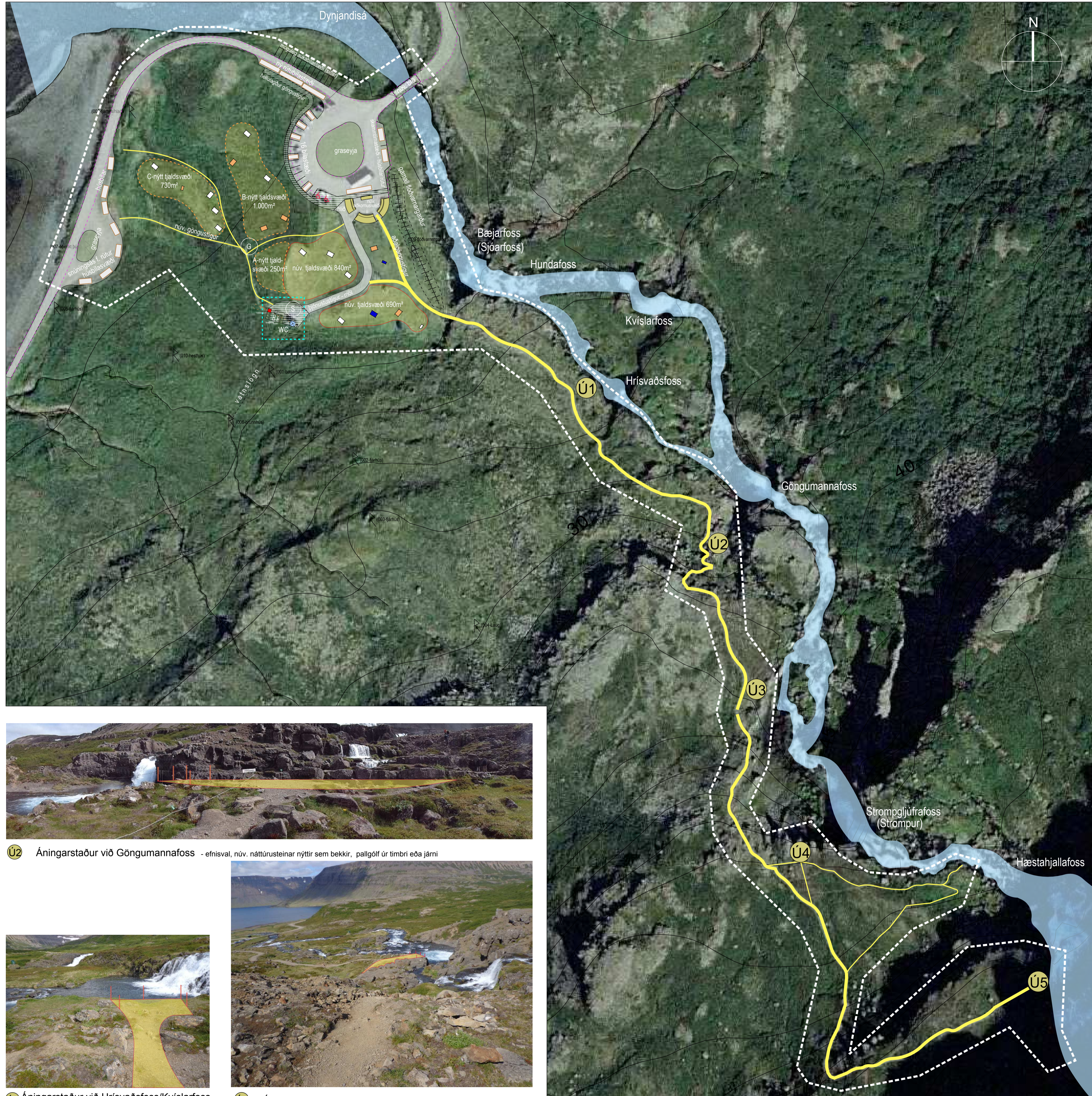
Ú1 Áningarstaður við Hrísvaðsfoss/Kvíslarfoss - aðstaða f. hreyfihamaða (m.a. umferð hjólastóla) - efnisval, pallgölf úr timri eða járn og létt öryggishandrið
